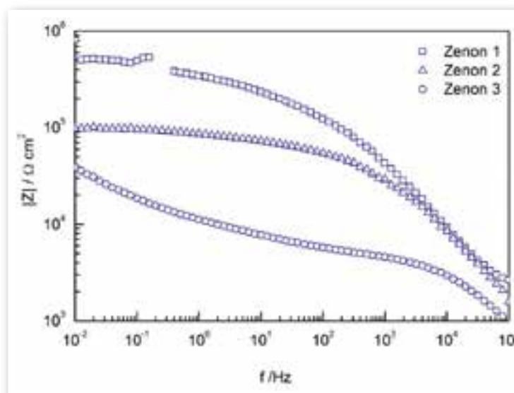
Figura 2. Evaluación de la corrosividad de las vitrinas de la sala de Egipto del Museo Arqueológico Nacional (Proyecto Air-Arte).
